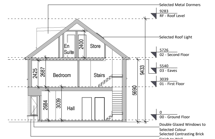
8 Section 1 1 : 200
