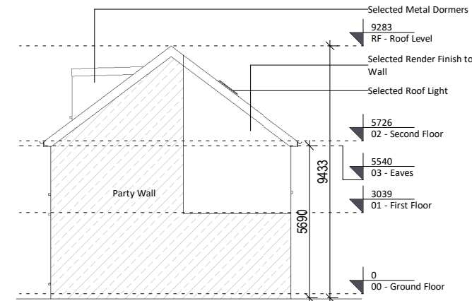
7 Right Elevation 1 : 200
