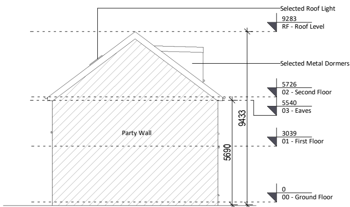
6 Left Elevation 1 : 200
